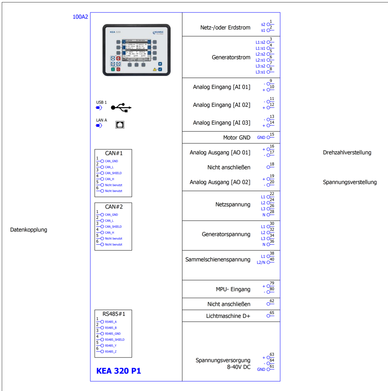
Abb. 6: Anschlussplan 1 der KEA 320 RP/KEA 320(-LT)
