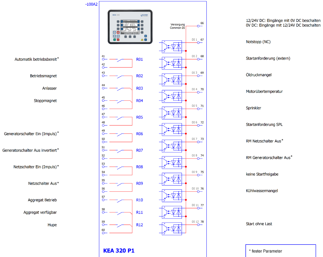
Abb. 7: Anschlussplan 2 der KEA 320 RP/KEA 320(-LT)
