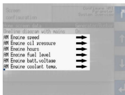
Abb. 9: AnalogManager für „Motor“ Werte in der Startseite
